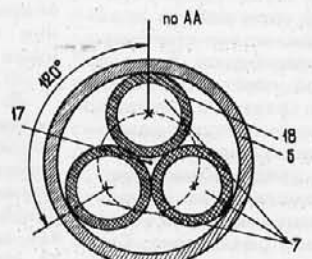
РИС. 3. Тубус фотоувеличителя (сечение по АА): 5 — тубус; 7 — световоды; 17 — оптическая ось фотоувеличителя; 18 — кожух световода
