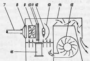
РИС. 4. Осветительный блок: 7 — световоды; 8 — зональный светофильтр; 9 — конденсор для лампы; 10 — лампы; 11 — световая заслонка; 12 — тепловой фильтр; 13 — отражатель; 14 — корпус осветительного блока; 15 — вентилятор; 16 — соленоид. Стрелками показана циркуляция воздуха
